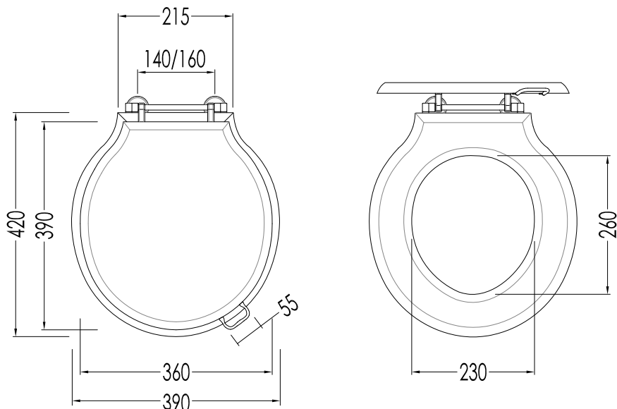
1. SEDILE LEGNO MASSELLO SOLID WOOD SEAT
