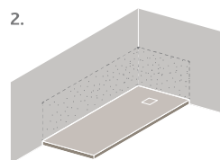
2. Posa del piatto doccia Shower tray installation Installation du receveur de douche
