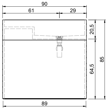
Prospetto frontale Front elevation
