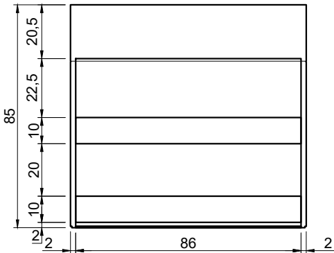
Prospetto posteriore Back elevation
