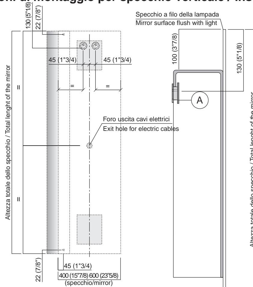
Fig. 2 Posizioni punti di fissaggio Location of fixing points
