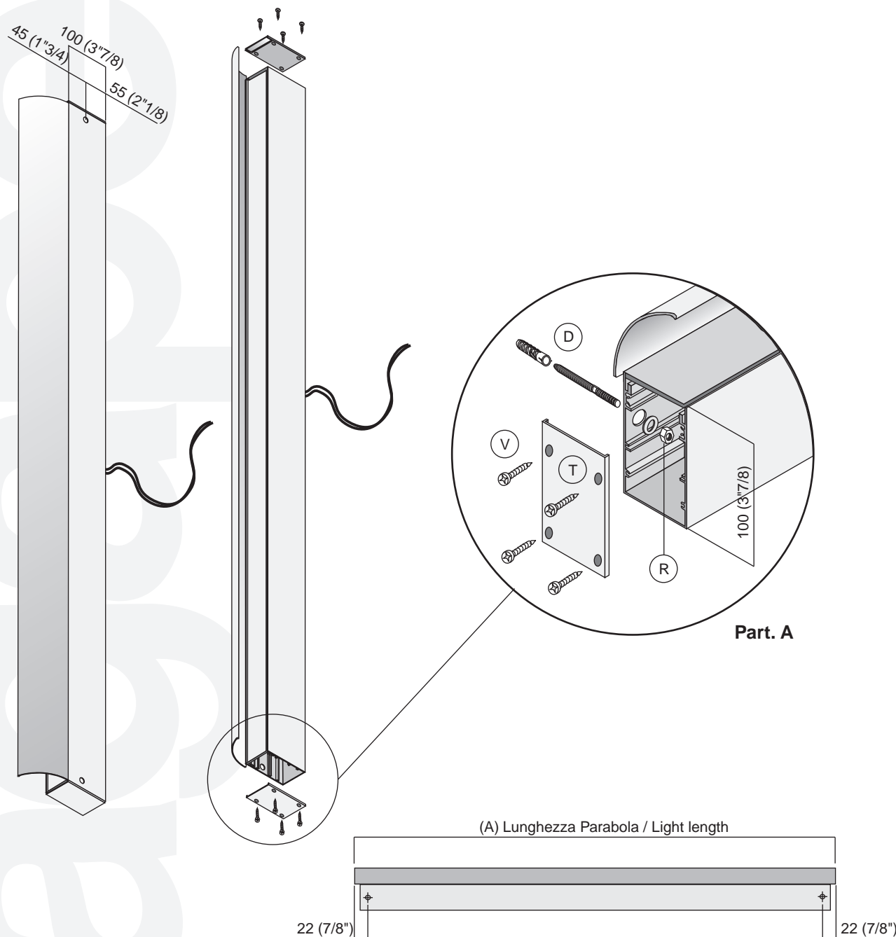
Fig. 1 Posizioni punti di fissaggio / Location of fixing points
