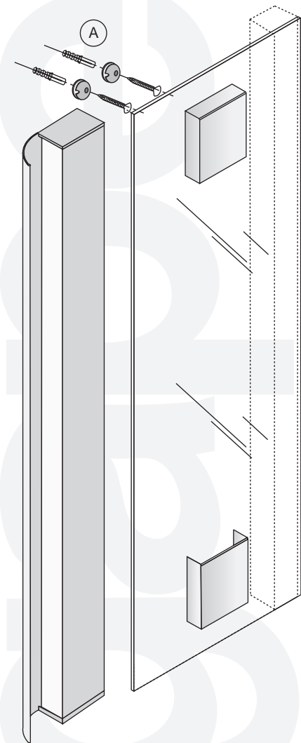
Fig. 2 Posizioni punti di fissaggio Location of fixing points
